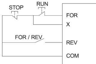
Трёхпроводной режим
